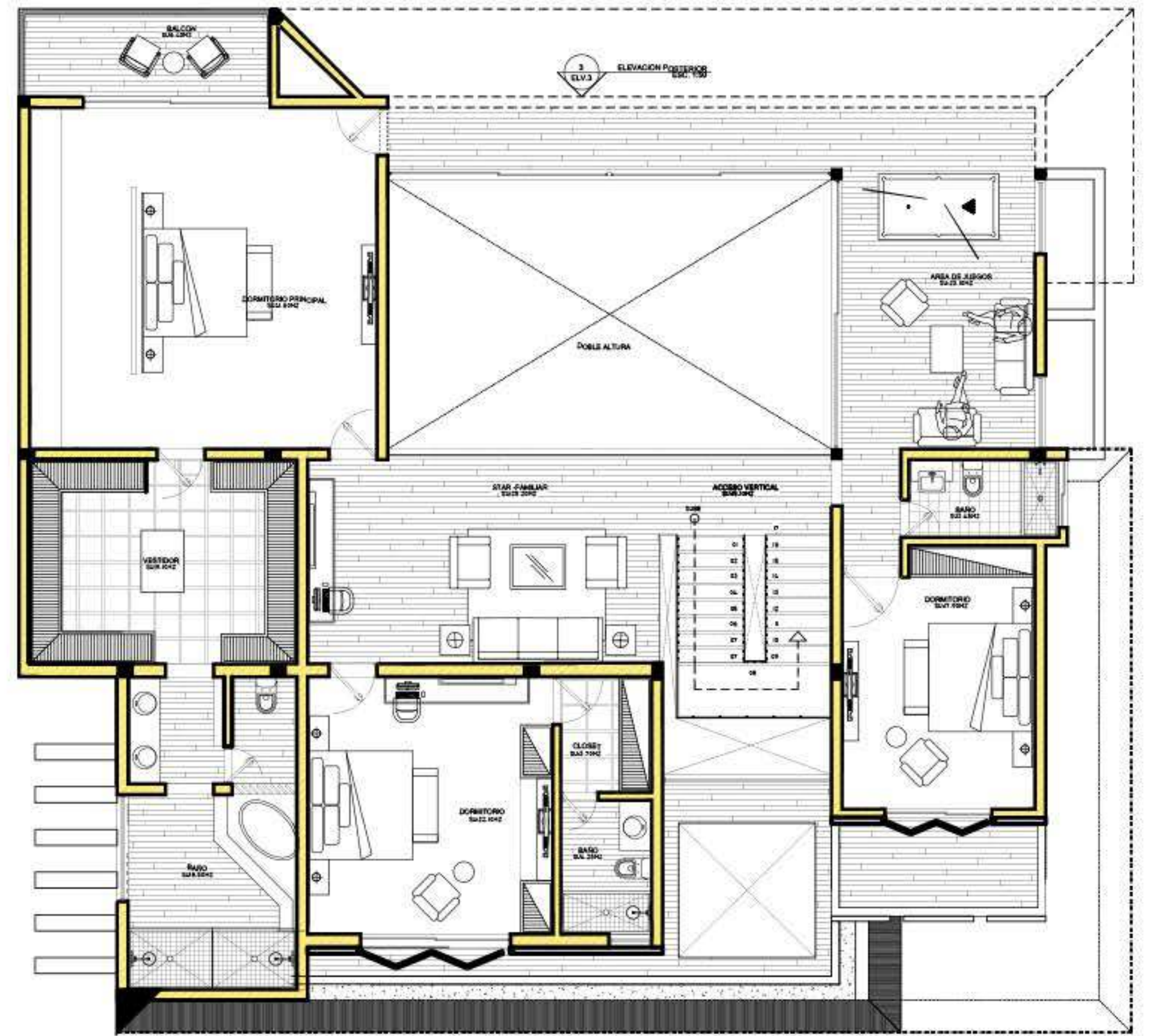
ARQ.#1 NIVEL 2 PLANTA ARQUITECTONICA 2DO NIVEL 2-NIVEL ESC. 1:50
