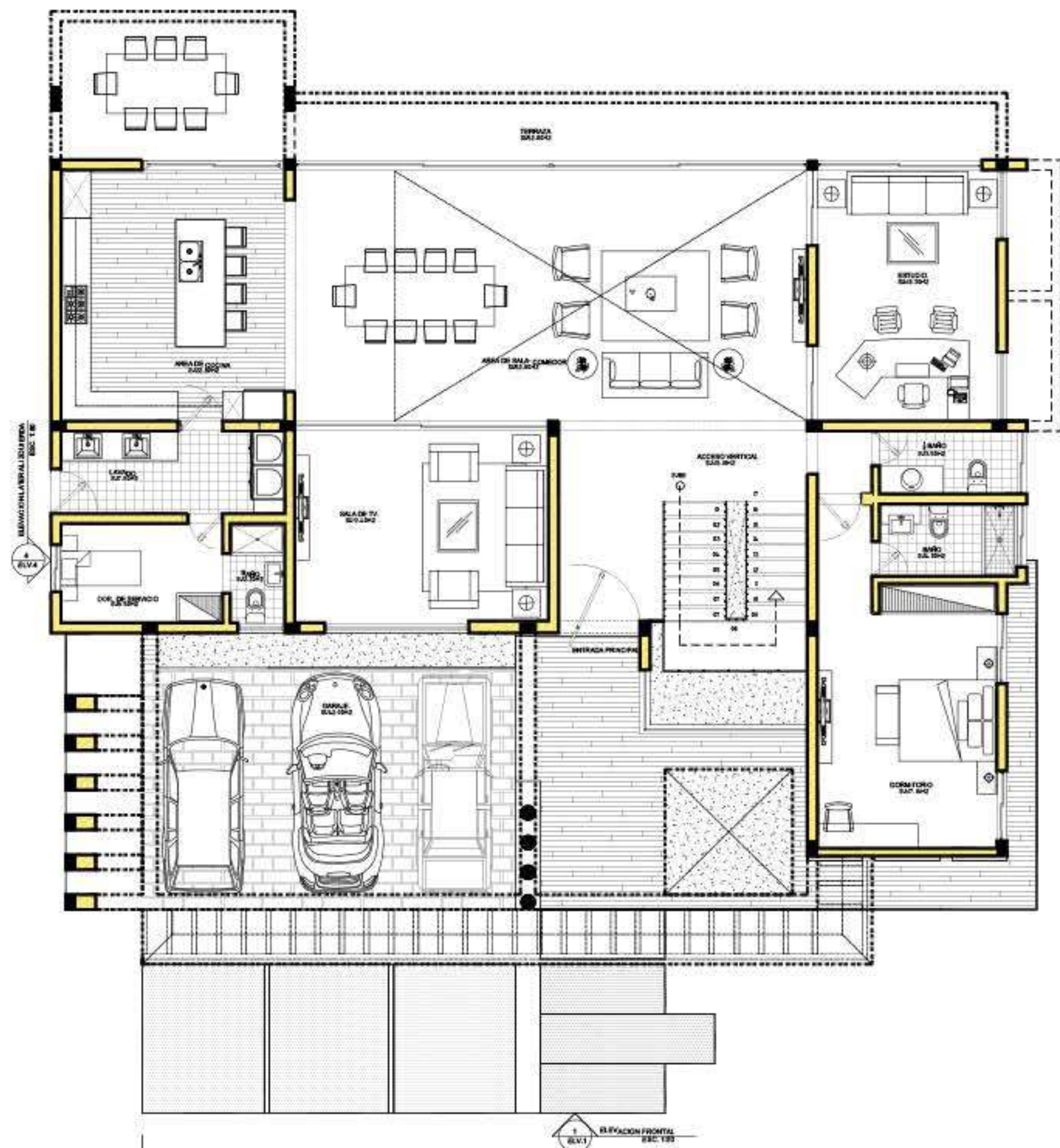
ARQ.#1 NIVEL 2 PLANTA ARQUITECTONICA 1ER NIVEL 2-NIVEL ESC. 1:50
